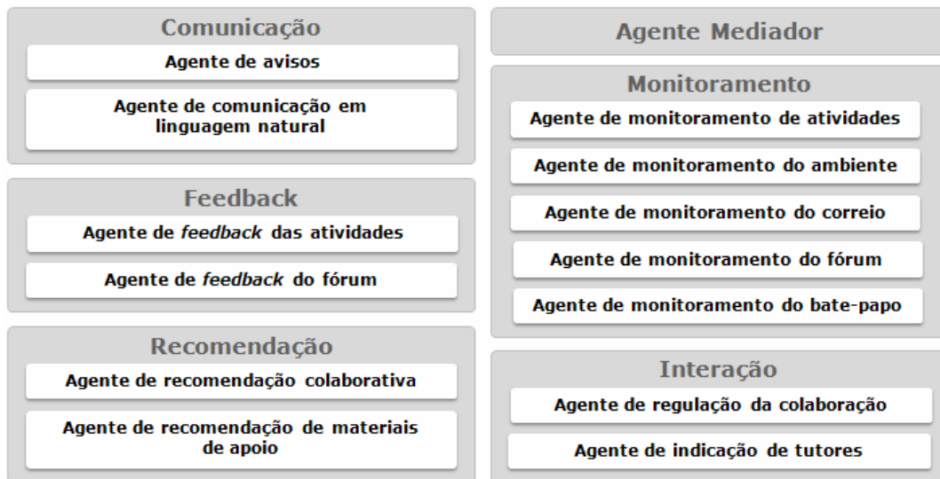
Figura 1: Componentes do sistema multiagente
